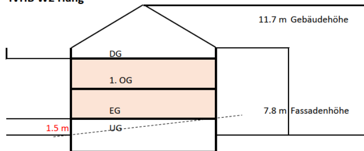
Abb. 42: Visualisierung der bestehenden Bestimmung und der Umsetzung durch die IVHB (Quelle: Jermann AG)
